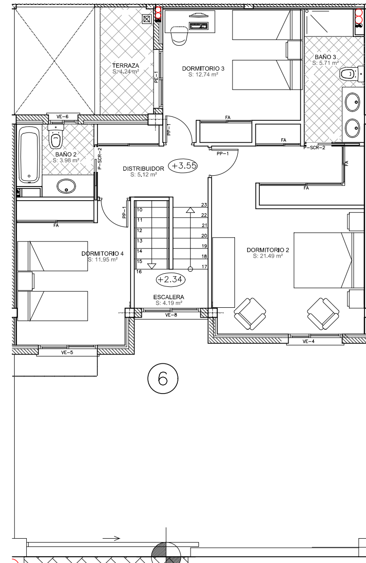
PLANTA PRIMERA
