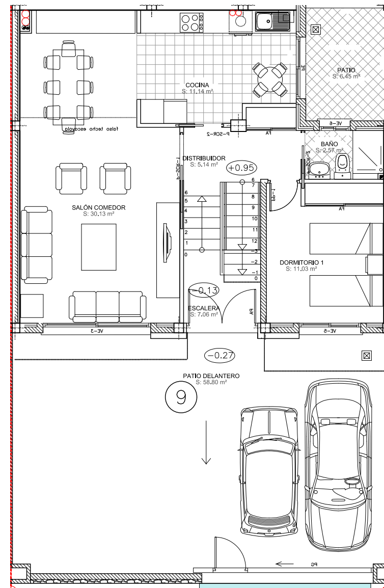
PLANTA BAJA
