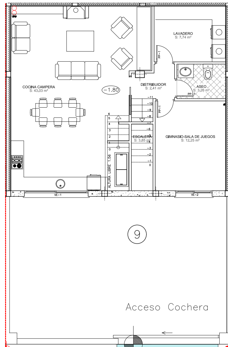
PLANTA SÓTANO
